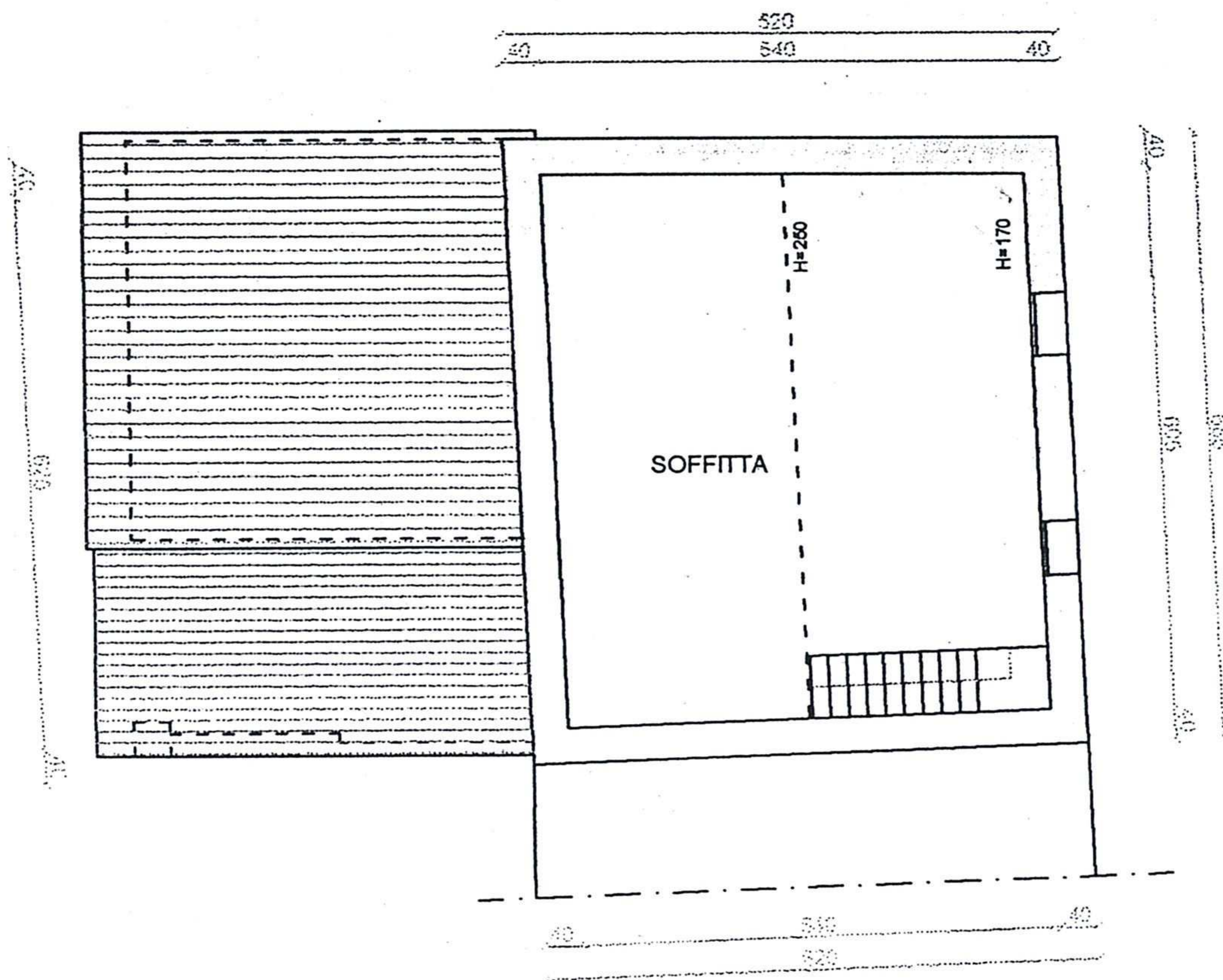
PIANTA PIANO SECONDO
